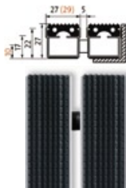
G Gummi-inlägg
